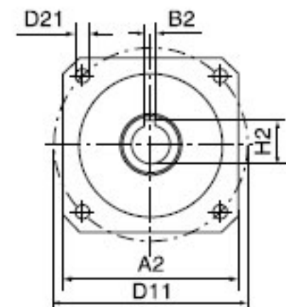
input 鍵槽型輸入 客戶要求
