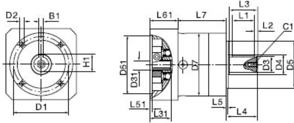
Other shaft 用戶可選擇的輸出類型
