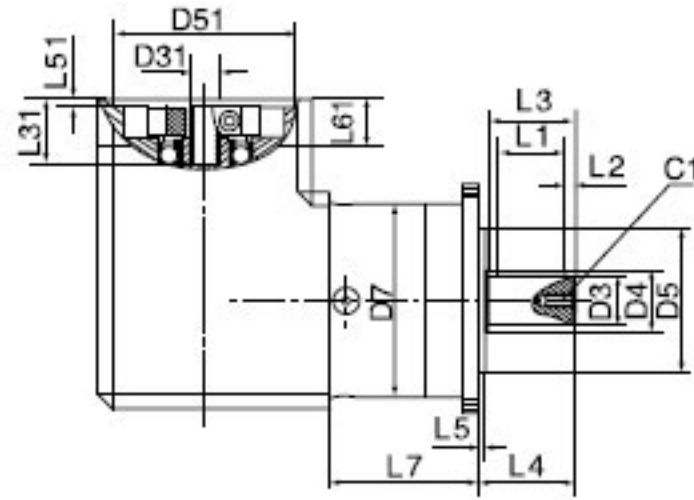
input 鎖緊環輸入 PF40-160標準
