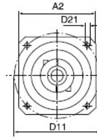
input 鎖緊環輸入 PL40-200標準
